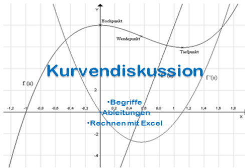
Abbildung 4: PPP-Kurvendiskussion
