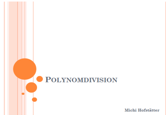
Abbildung 13: PPP-Polynomdivisionen
