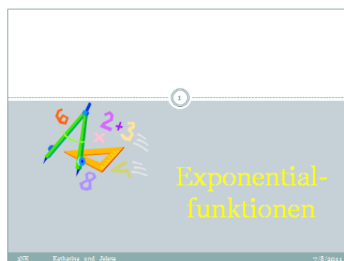
Abbildung 3: PPP-Exponentialfunktionen
