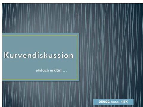
Abbildung 2: PPP-Kurvendiskussion
